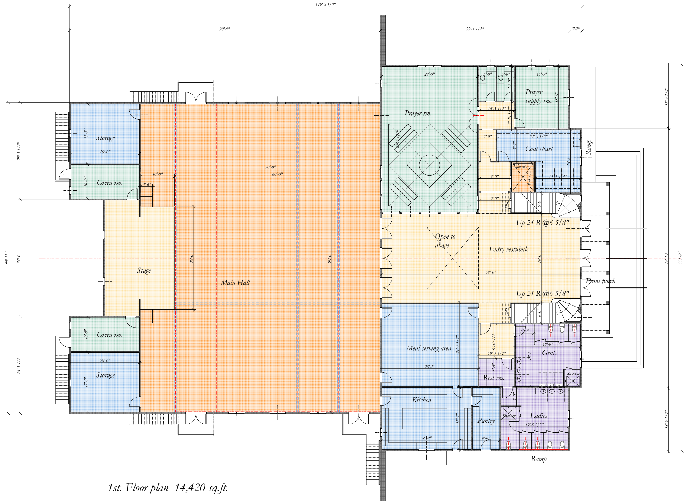
Scale 1/16"=1'-0"
